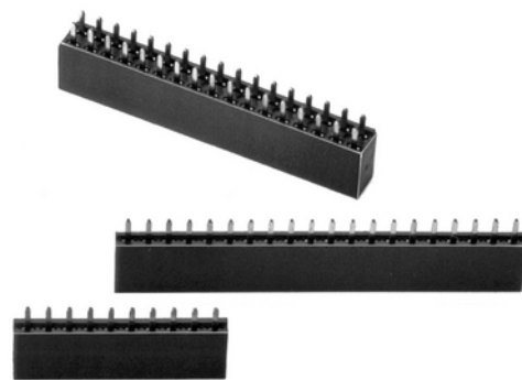
Gabelkontakte für Vierkantstifte 0,635mm. Fork contacts accept 0.635mm square pins.
