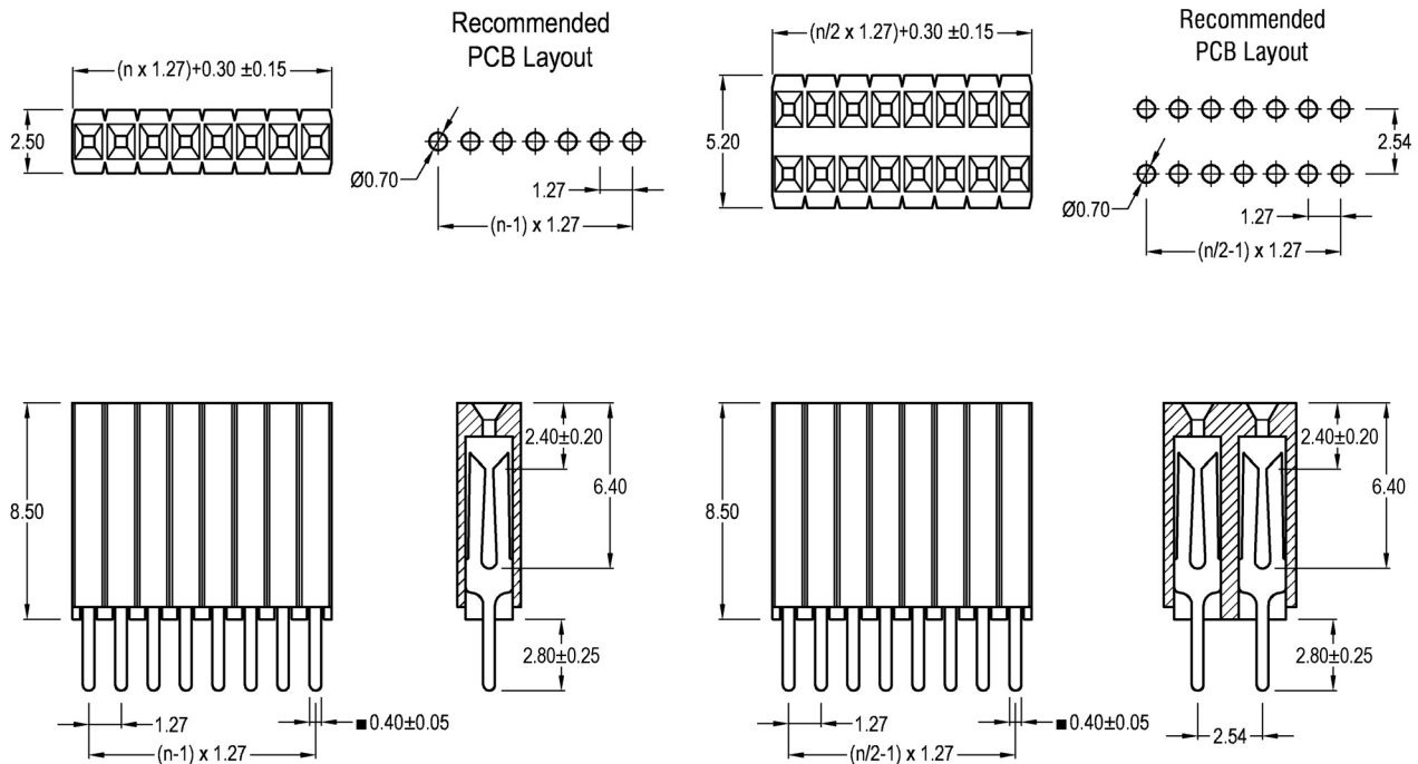
Gabelkontakte für Vierkantstifte 0,46mm. Fork contacts accept 0.46mm square pins.
