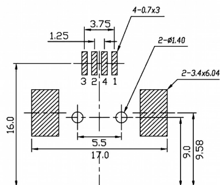
PCB EDGE PCB LAYOUT (COMPONENT SIDE)
